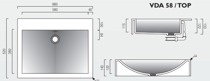
VDA 58 / TOP
